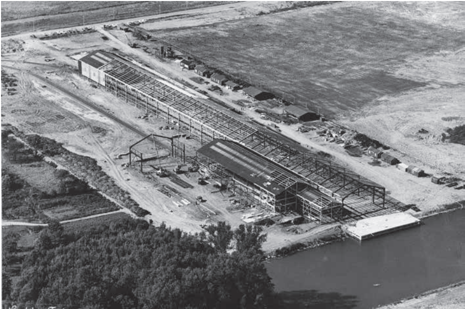
In de zomer van 1964 was de bouw van de nieuwe fabriek al een eind op streek. Op 31 december 1964 zou hier de eerste buis worden getrokken. Twee jaar later werd de fabriek al verkocht.
