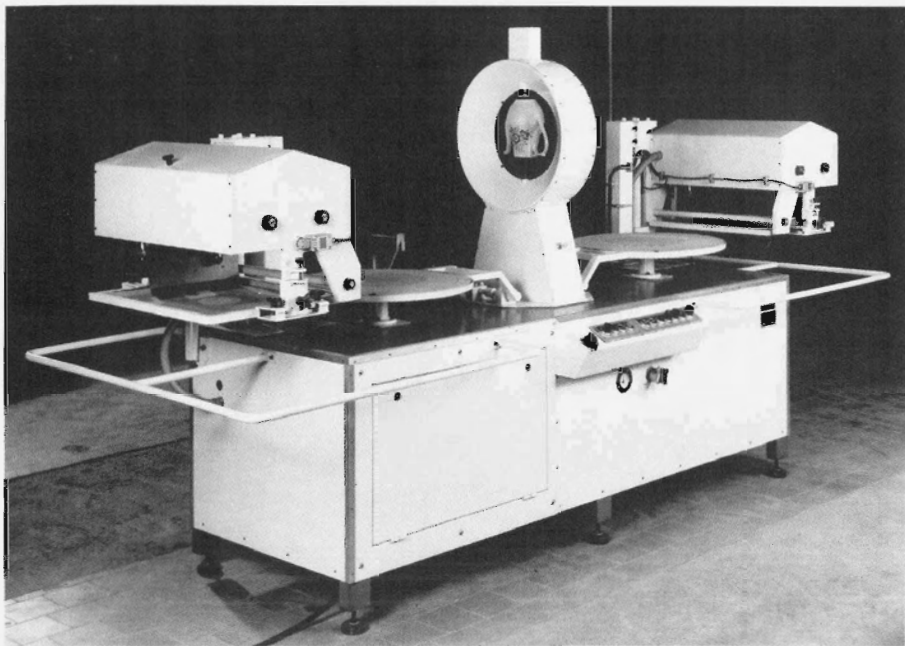
De vacuüm-silkscreenmachine was speciaal ontworpen om decors via de zeefdruktechniek aan te brengen op bolle voorwerpen, zoals koffiepotten. Collectie SHCL, fotoarchief Sphinx-Céramique.
